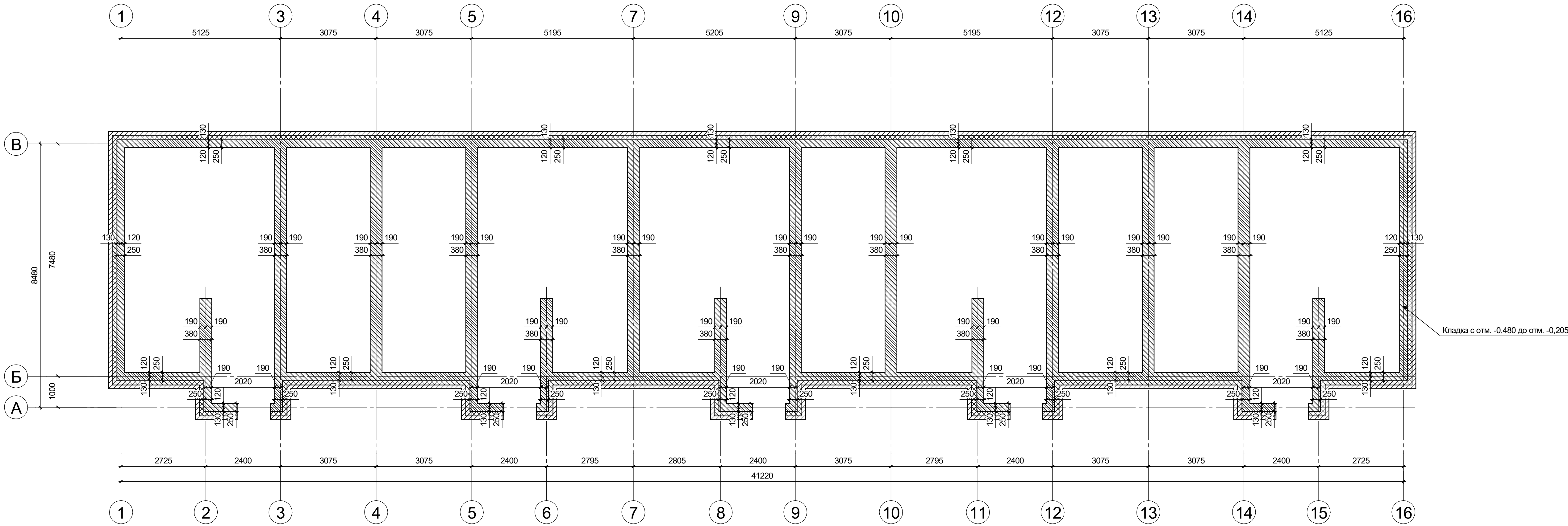
Кладочный план цоколя
