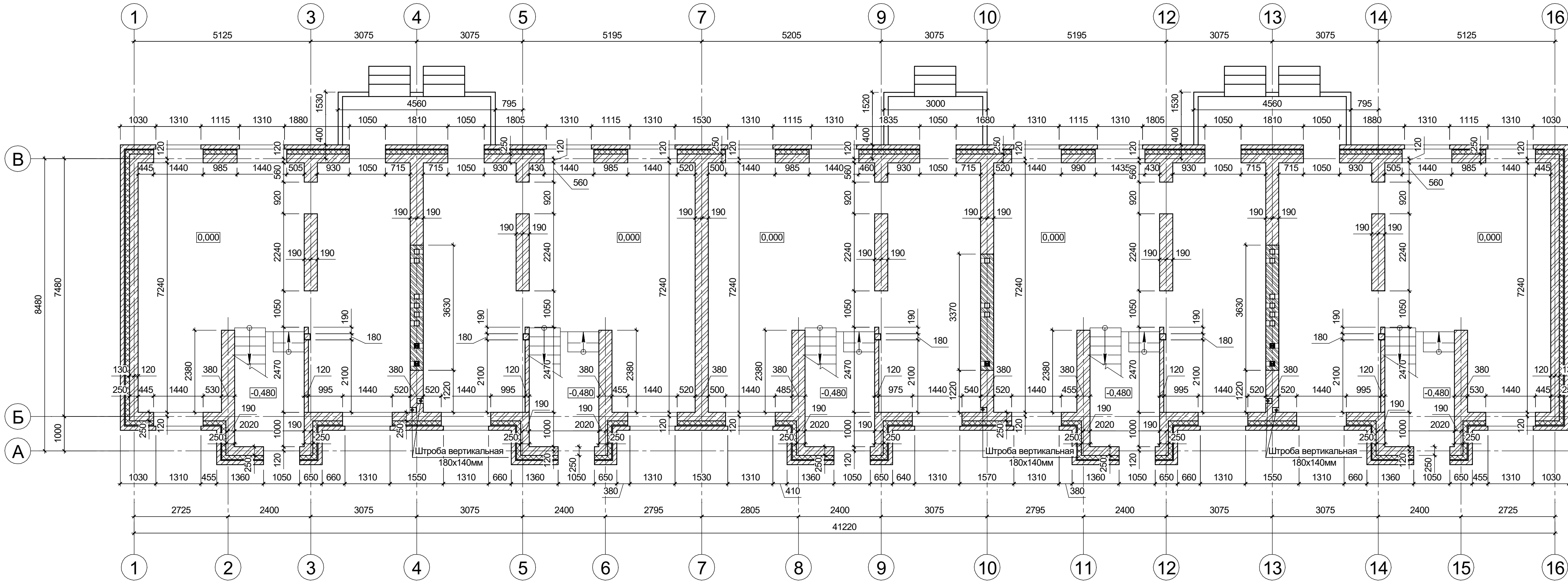
Кладочный план на отм. 0,000
