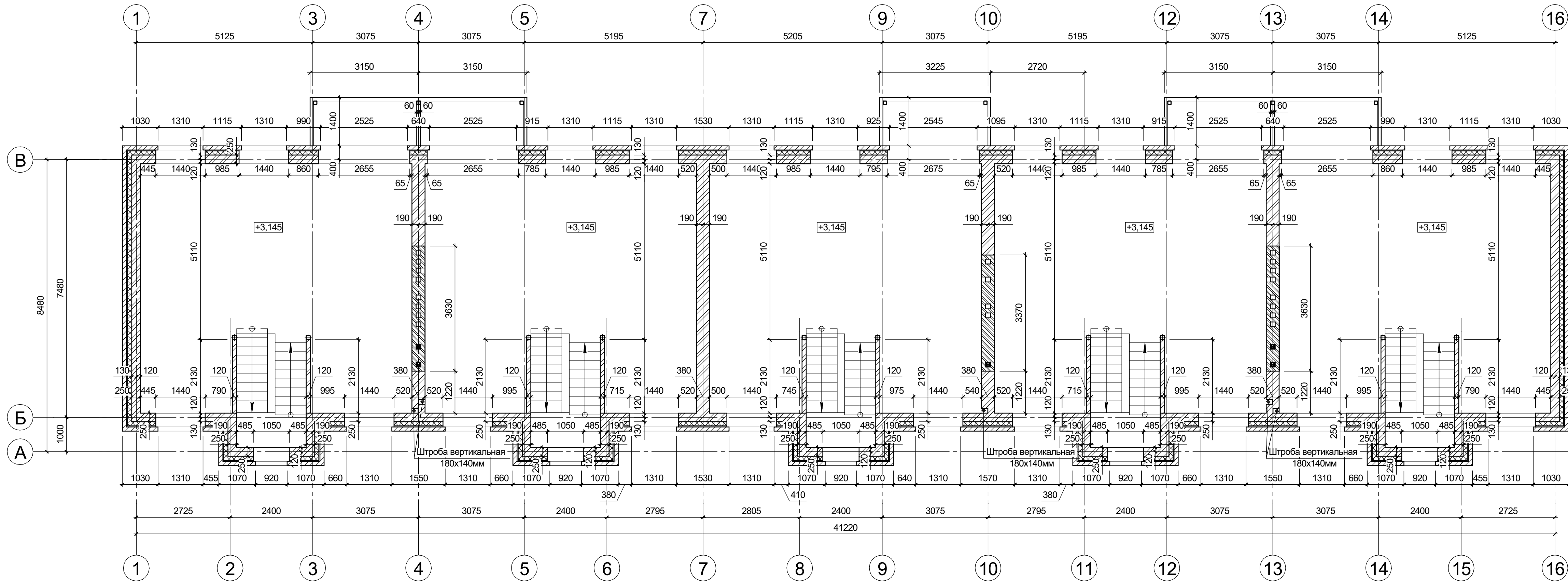
Кладочный план на отм. +3,145
