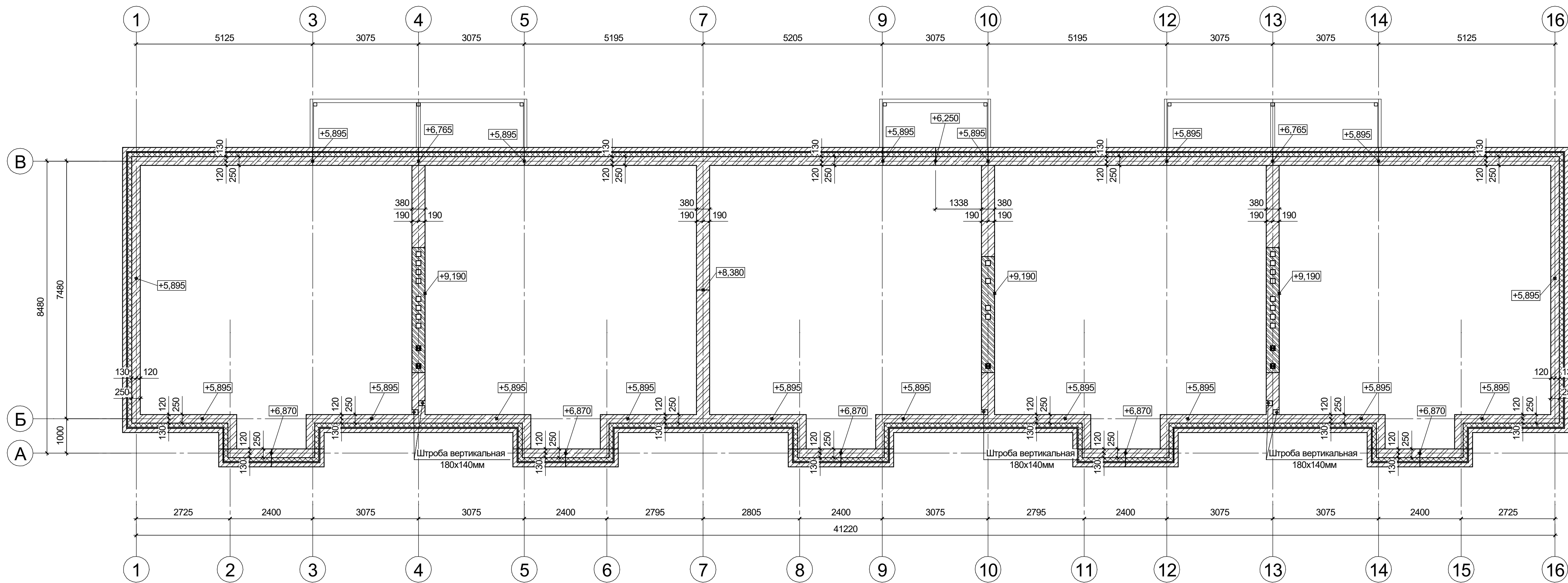
Кладочный план на отм. +5,895
