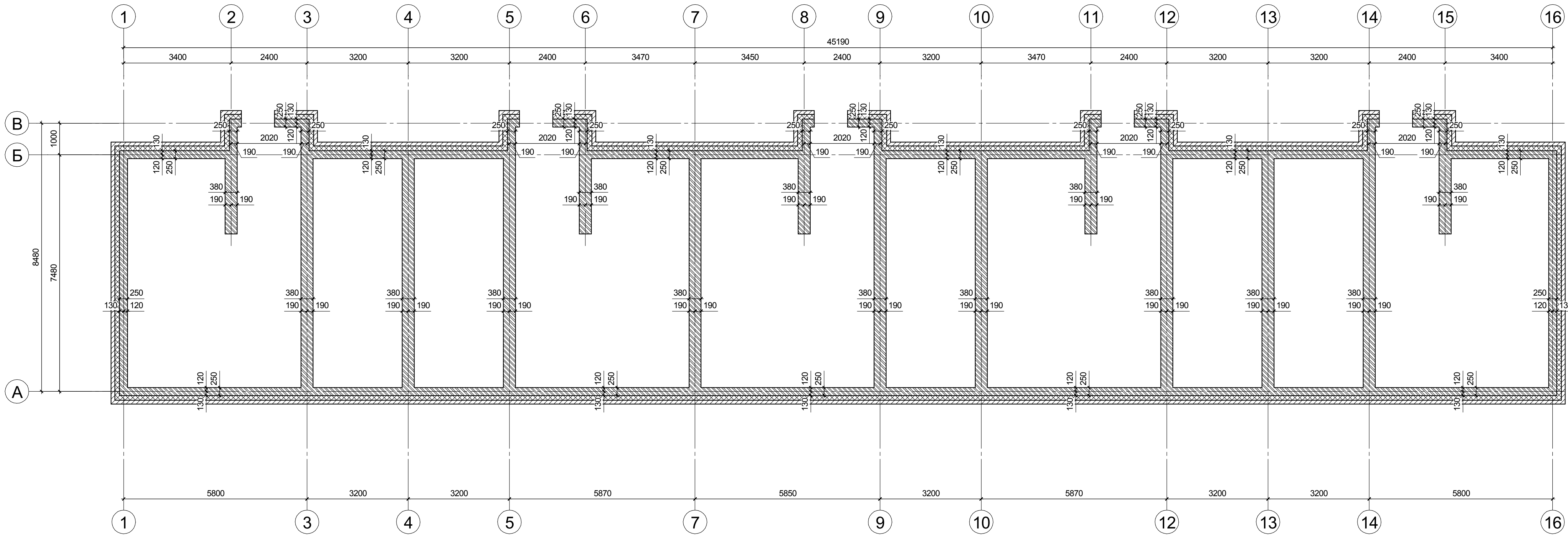
Кладочный план на отм. 0.000
