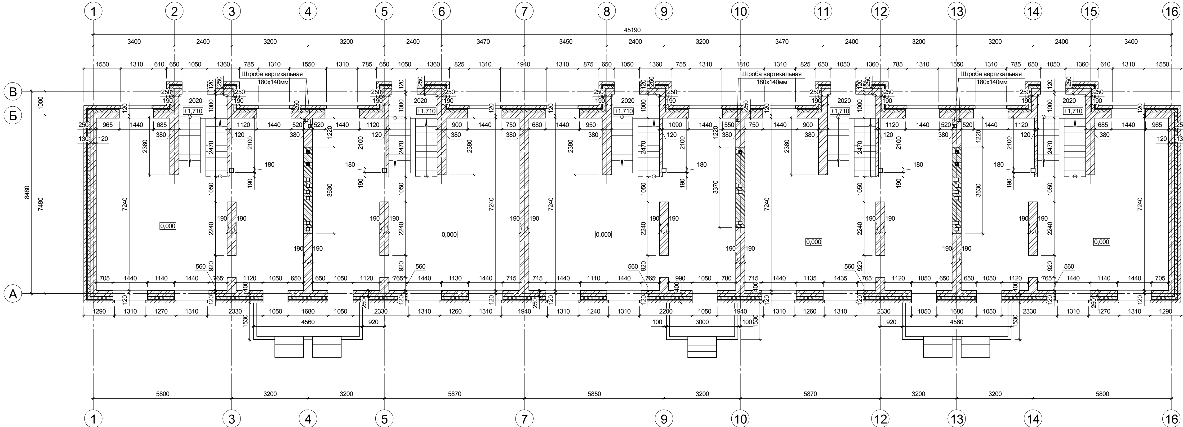
Кладочный план на отм. 0.000
