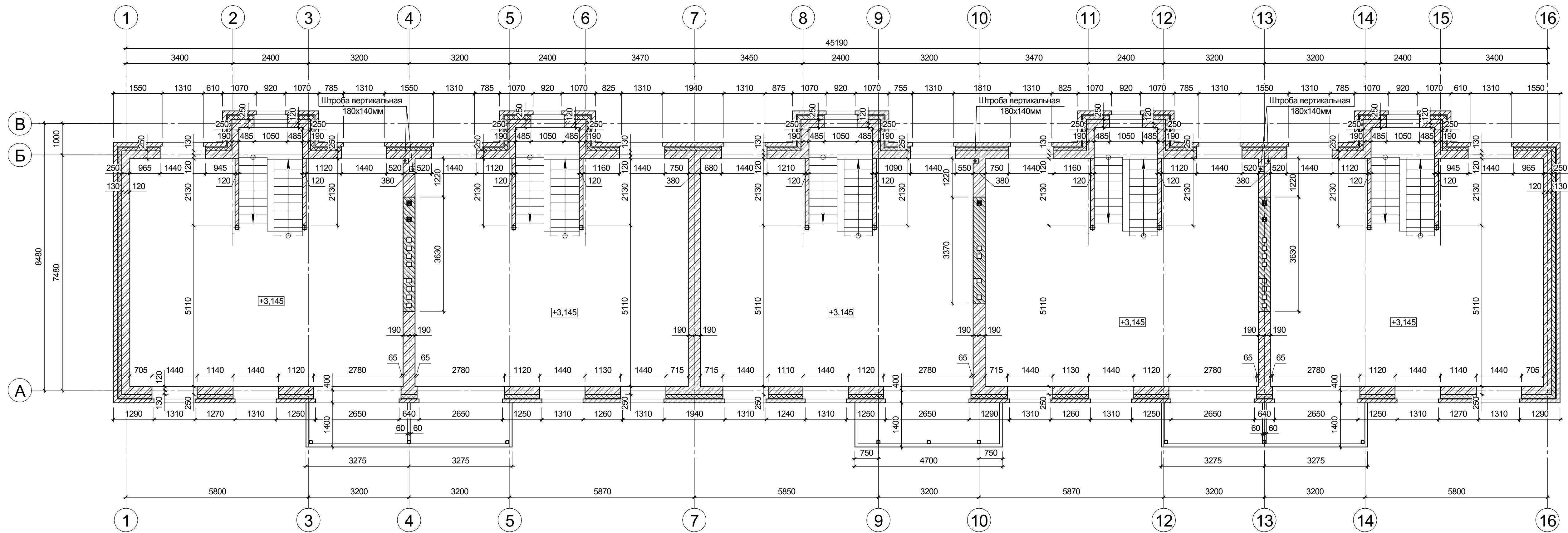
Кладочный план на отм. +5,895
